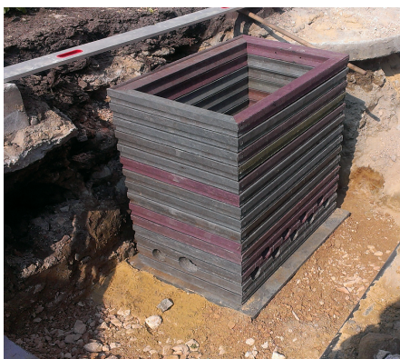
Jednoduchá instalace komory díky modulárnímu systému skládaných dílů - bez nutnosti lepení nebo betonáže.
